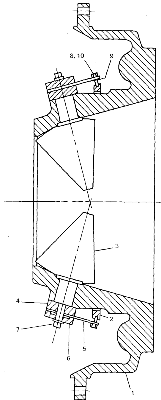
FIG. 7— PRV ASSEMBLY
