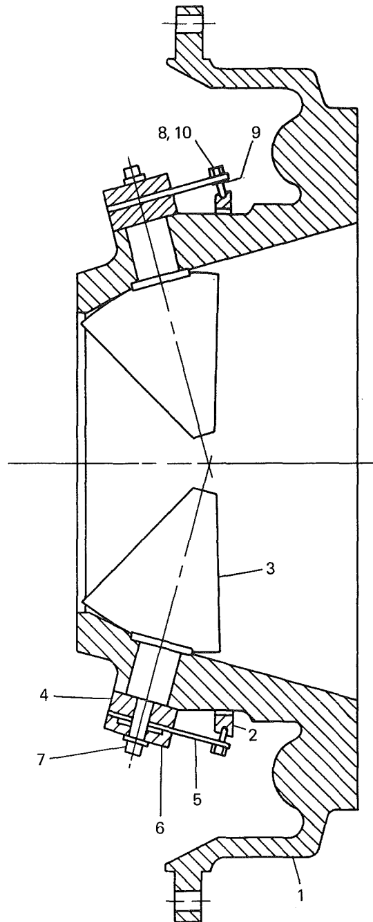
FIG. 7- PRV ASSEMBLY
