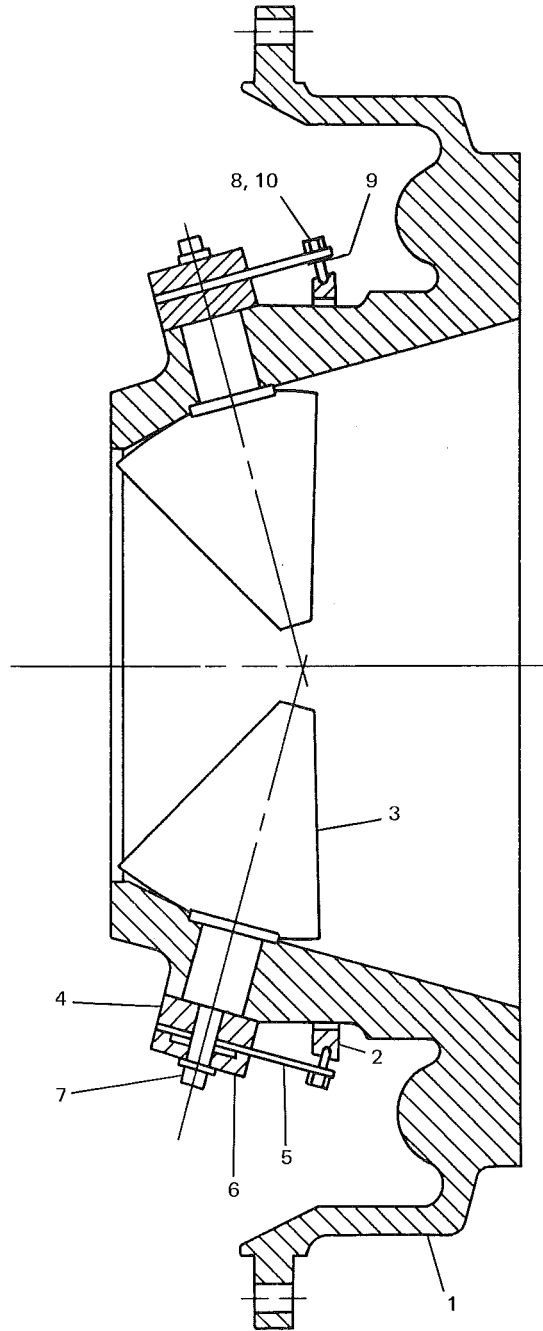
FIG. 12— PRV ASSEMBLY
