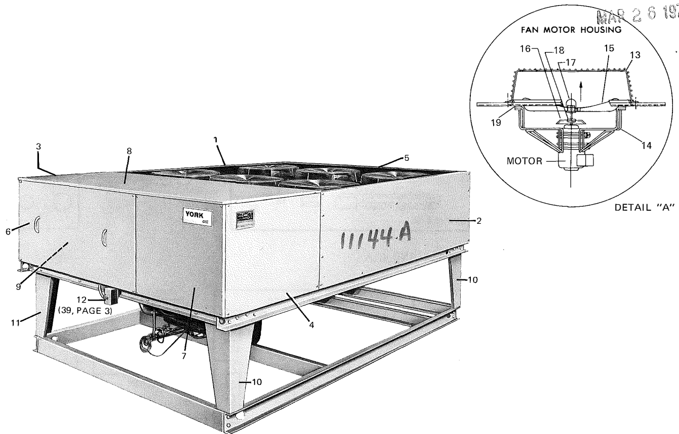
FIG. 1—MODEL LCHA45
