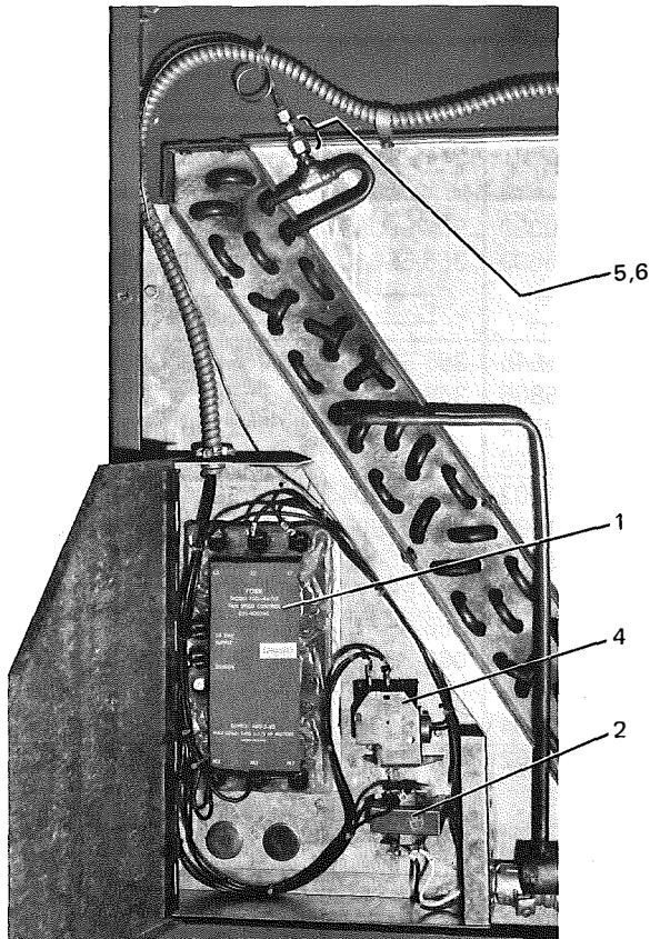
FIG. 5 - FAN SPEED CONTROL
