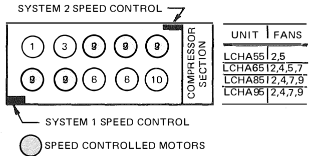
FIG. 6 - FAN MOTOR LOCATION
